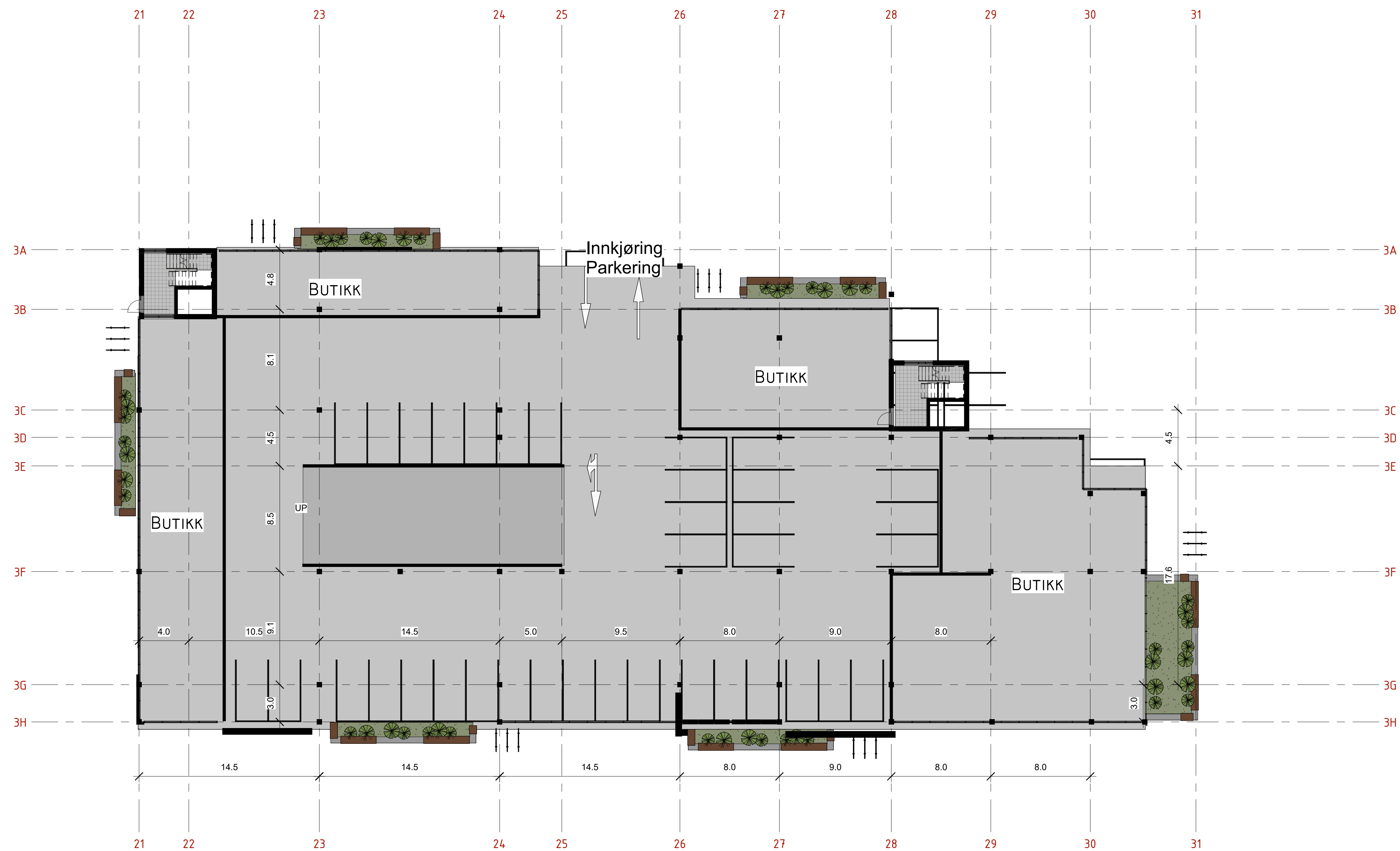
Plan 01 - Sørlig kvartal 1:200
