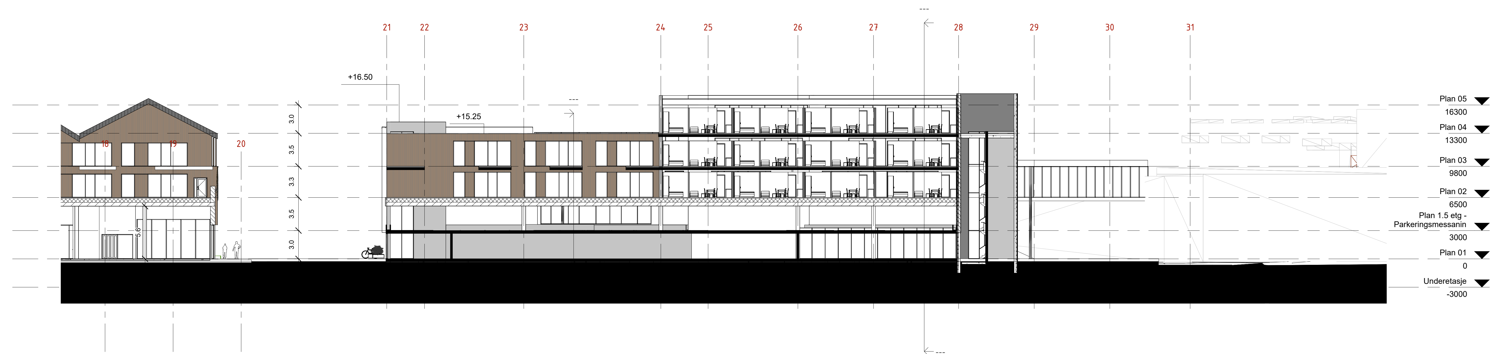
Snitt A-A - Dependent 2 1:200
