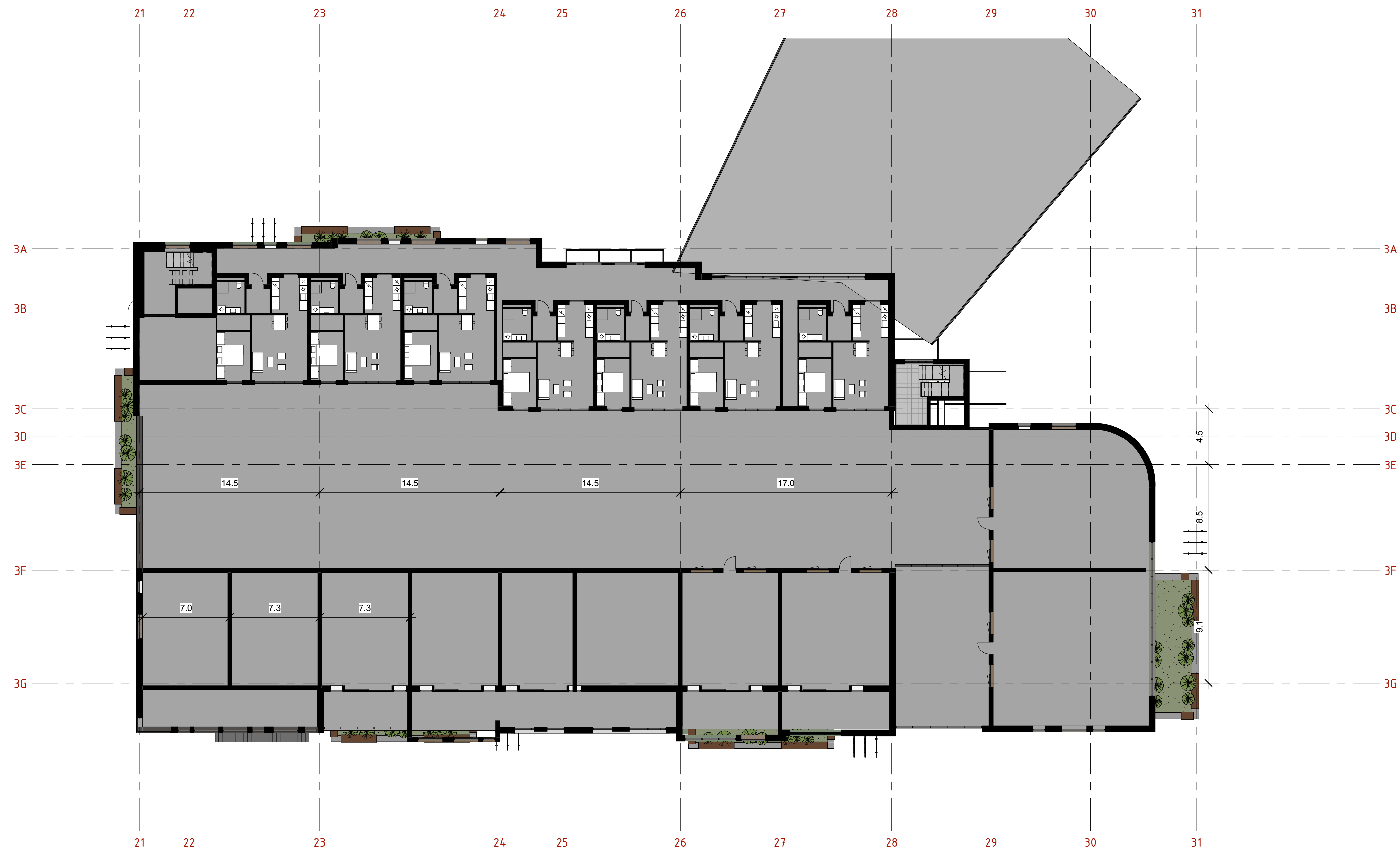
Plan 02 - Sørlig kvartal 1 : 200
