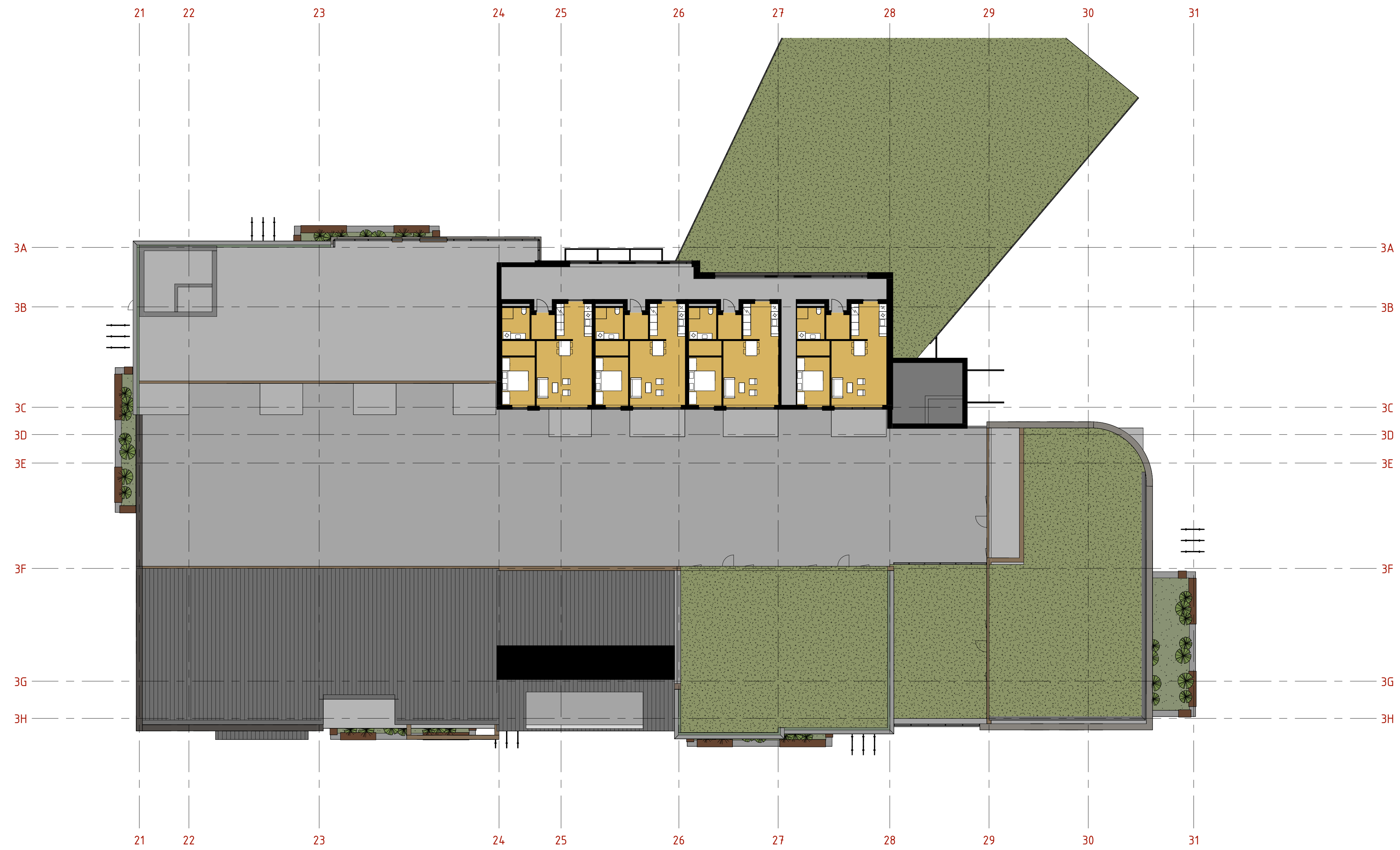
Plan 04 - Sørlig kvartal 1 : 200
