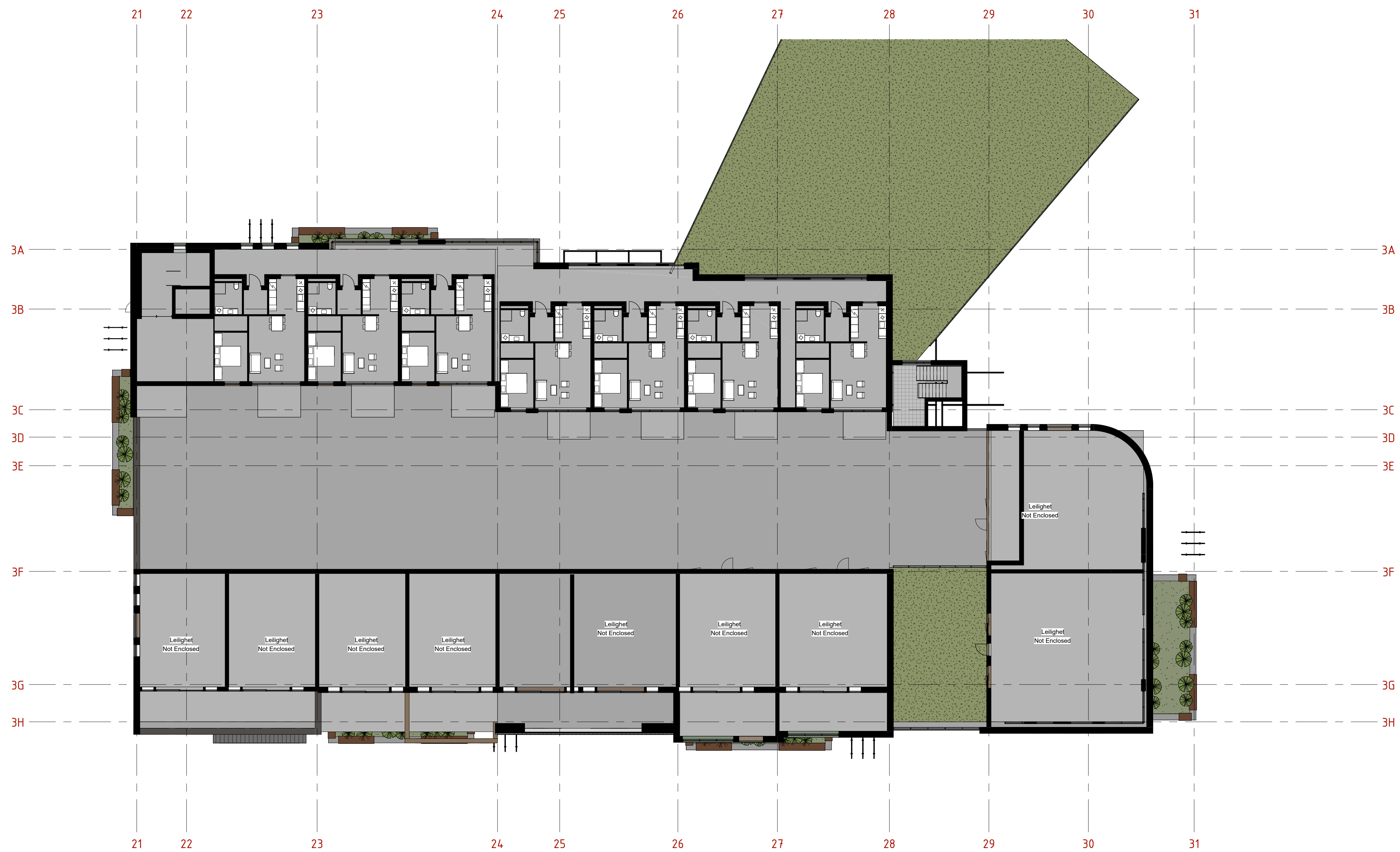
Plan 03 - Sørlig kvartal 1:200
